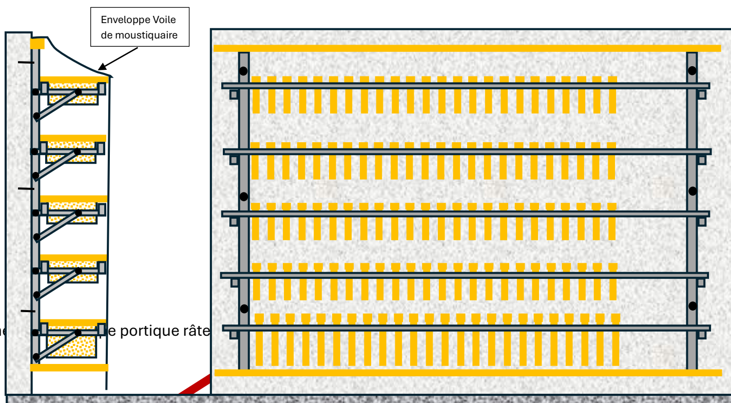
B – Schéma de principe d'un portique fixé à un mur
