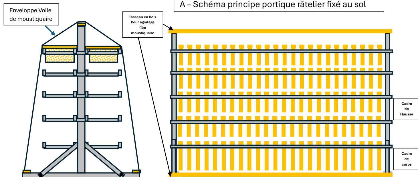
A – Schéma principe portique râtelier fixé au sol
